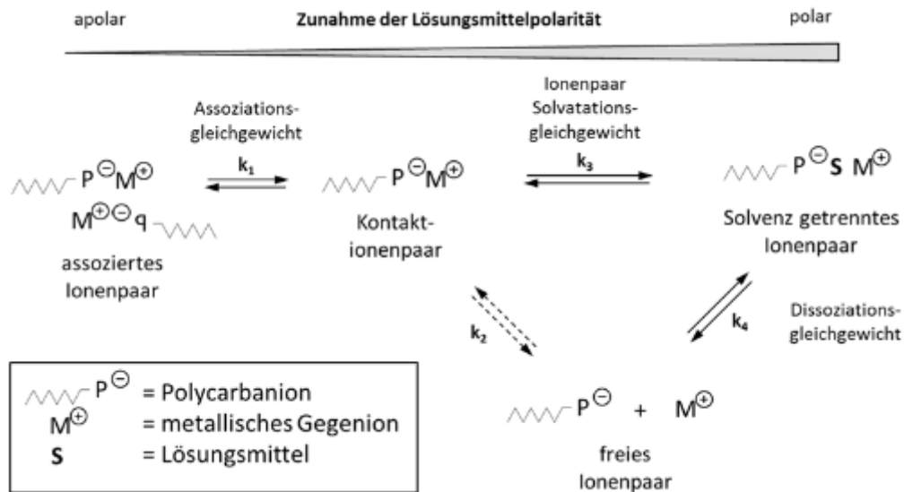
Abb. 1: Die Abbildung zeigt den Einfluss des Lösemittels auf das gleichgewicht der Ionen im falle der Anionischen Polymerisation. [1]
