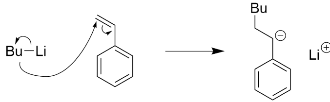
Abb. 2: Die Abbildung zeigt den Initiatorschritt von Styrol mit BuLi.
